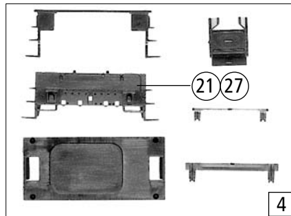
19 o. Abb. / no ill. Tenderleitung-Behälterl.Satz Tender line-box set
